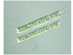
Melosira ambigua
